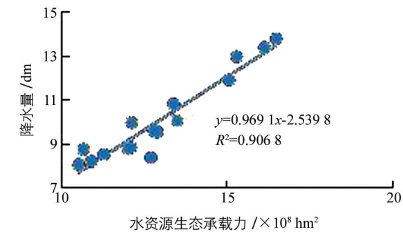
图 3 成都市降水量与水资源生态承载力相关关系
