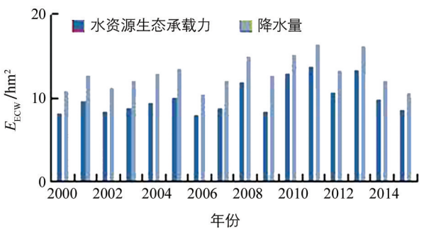
图 2 成都市历年水资源生态承载力与降水量
