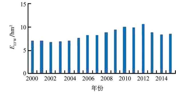
图 1 成都市历年水资源生态足迹
