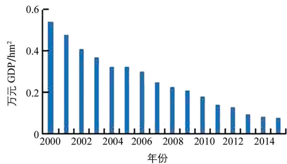
图 4 成都市历年水资源万元 GDP 生态足迹
