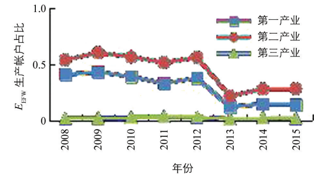
图 5 人均水资源生态足迹生产账户历年变化
