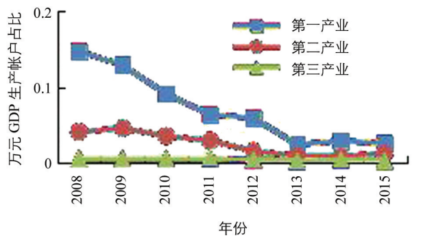
图 6 万元 GDP 生态足迹生产账户历年变化
