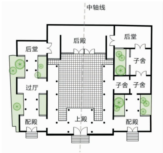
图 5 罗家祠堂平面图
