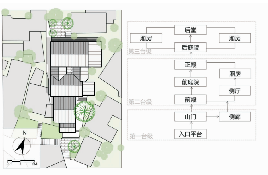
图 8 老官庙(古县衙)层级分析图(根据赵万民《松溉古镇》改绘)
